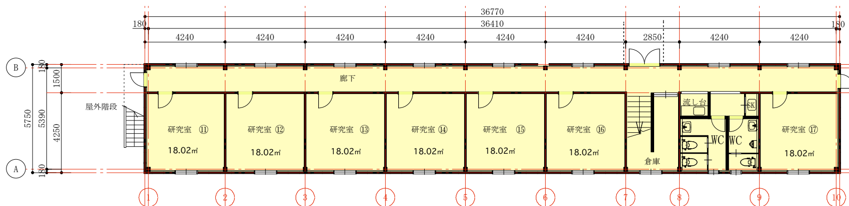
1階平面図
